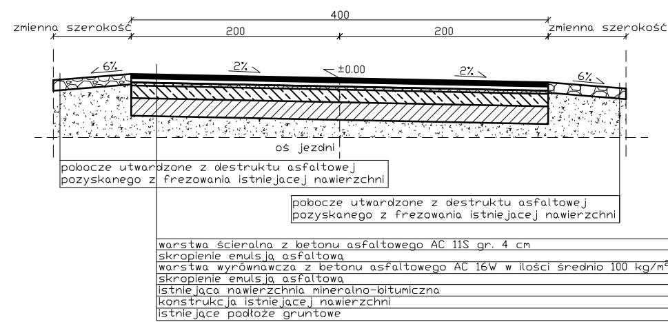
PRZEKRÓJ NORMALNY JEZDNI NA ŁUKU KOŁOWYM (WZMOCNIENIE ISTNIEJĄCEJ KONSTRUKCJI- SPADEK JEDNOSTRONNY)
