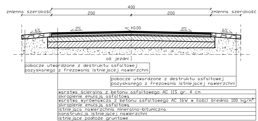
PRZEKRÓJ NORMALNY JEZDNI NA PROSTEJ-OBOWIĄZUJE DO KM 0+880,00 (WZMOCNIENIE ISTNIEJĄCEJ KONSTRUKCJI- SPADEK DASZKOWY)
