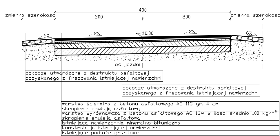
PRZEKRÓJ NORMALNY JEZDNI NA ŁUKU KOŁOWYM (WZMOCNIENIE ISTNIEJĄCEJ KONSTRUKCJI- SPADEK JEDNOSTRONNY)
