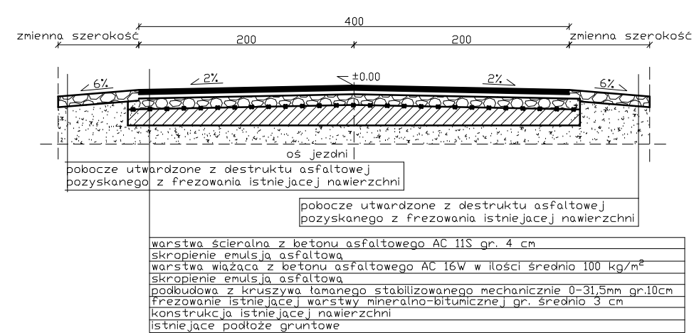
PRZEKRÓJ NORMALNY JEZDNI NA PROSTEJ KM DD 0+880,00 DO KM 2+529,92 (WZMOCNIENIE ISTNIEJĄCEJ KONSTRUKCJI- SPADEK DASZKOWY)
