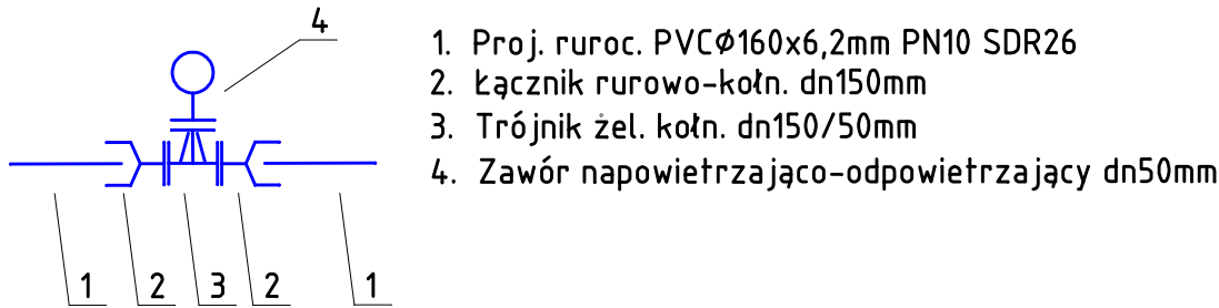
SCHEMAT WĘZŁA NR W42
