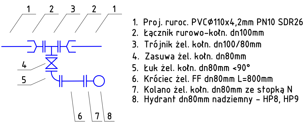
SCHEMAT WĘZŁA NR W63, W69
