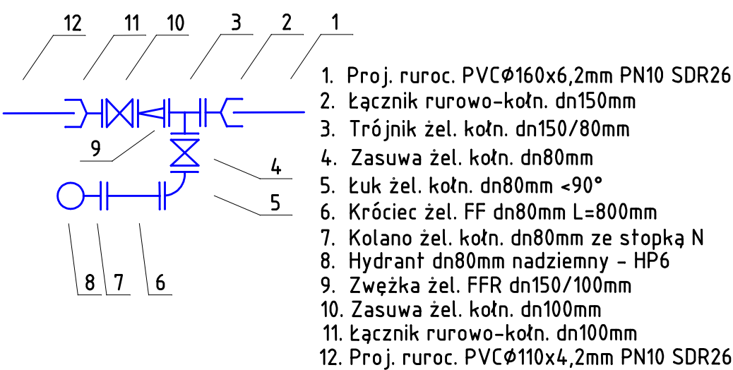
SCHEMAT WĘZŁA NR W47a
