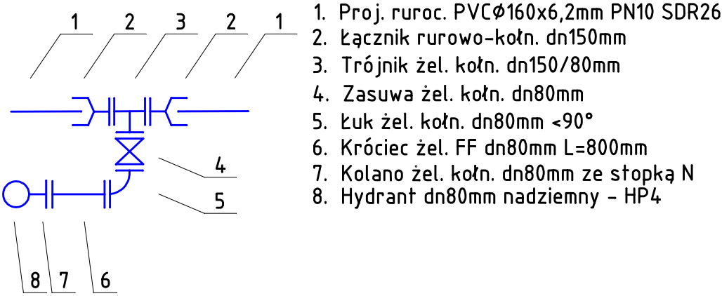
SCHEMAT WĘZŁA NR W37
