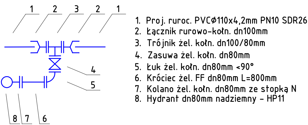
SCHEMAT WĘZŁA NR W84
