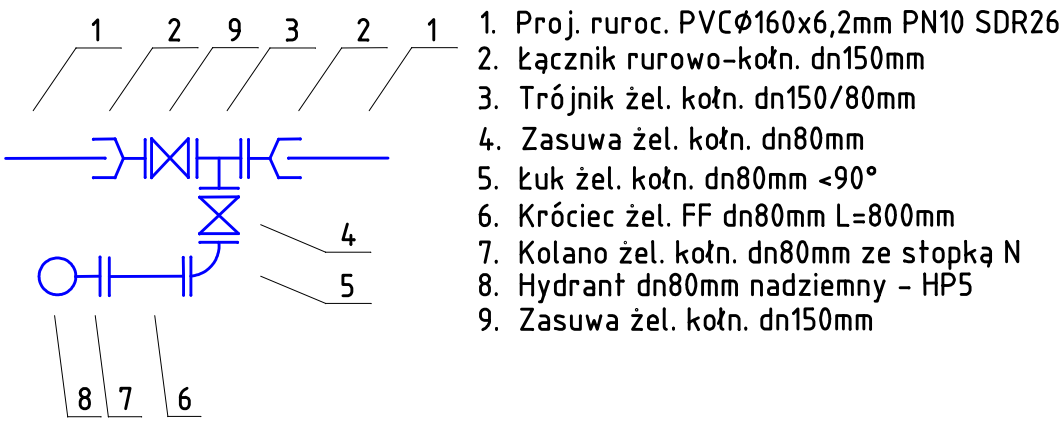
SCHEMAT WĘZŁA NR W44a
